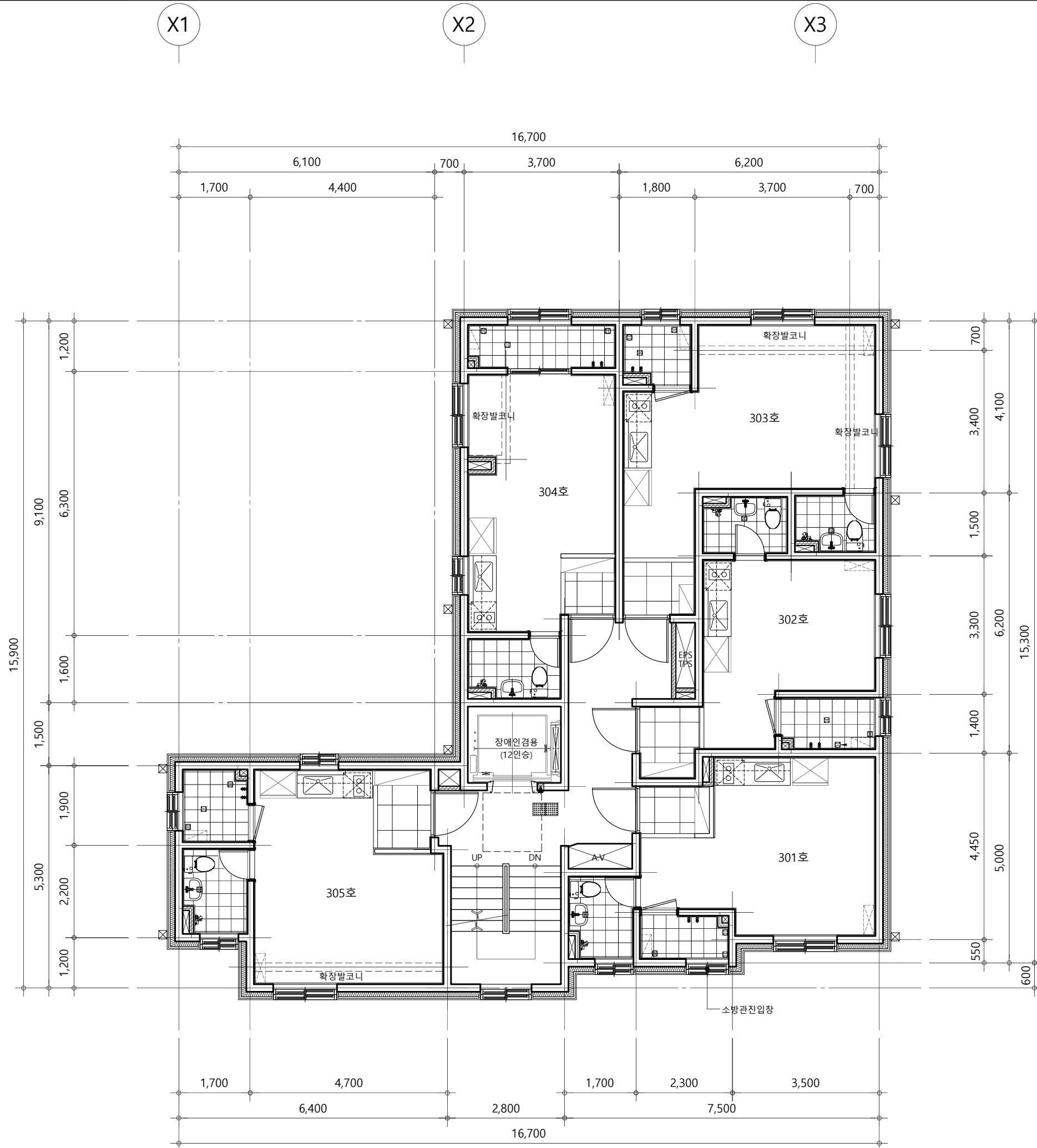
1 - 3층 평면도 1 : 100
